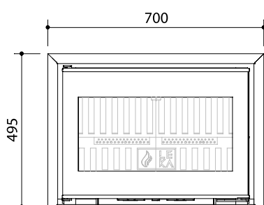
Profil 3 Côtés
