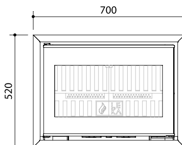
Profil 4 Côtés
