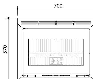
Profil 4 Côtés
